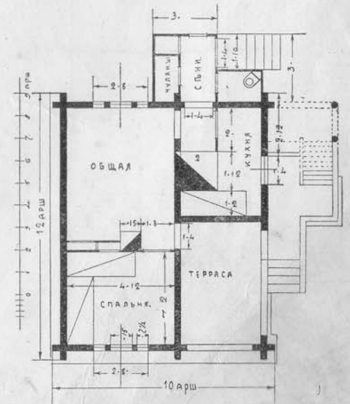
Планъ.
