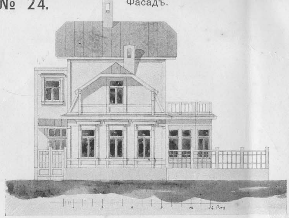
Фасадъ.
