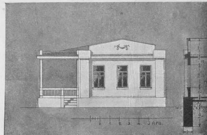
Фасадъ.
