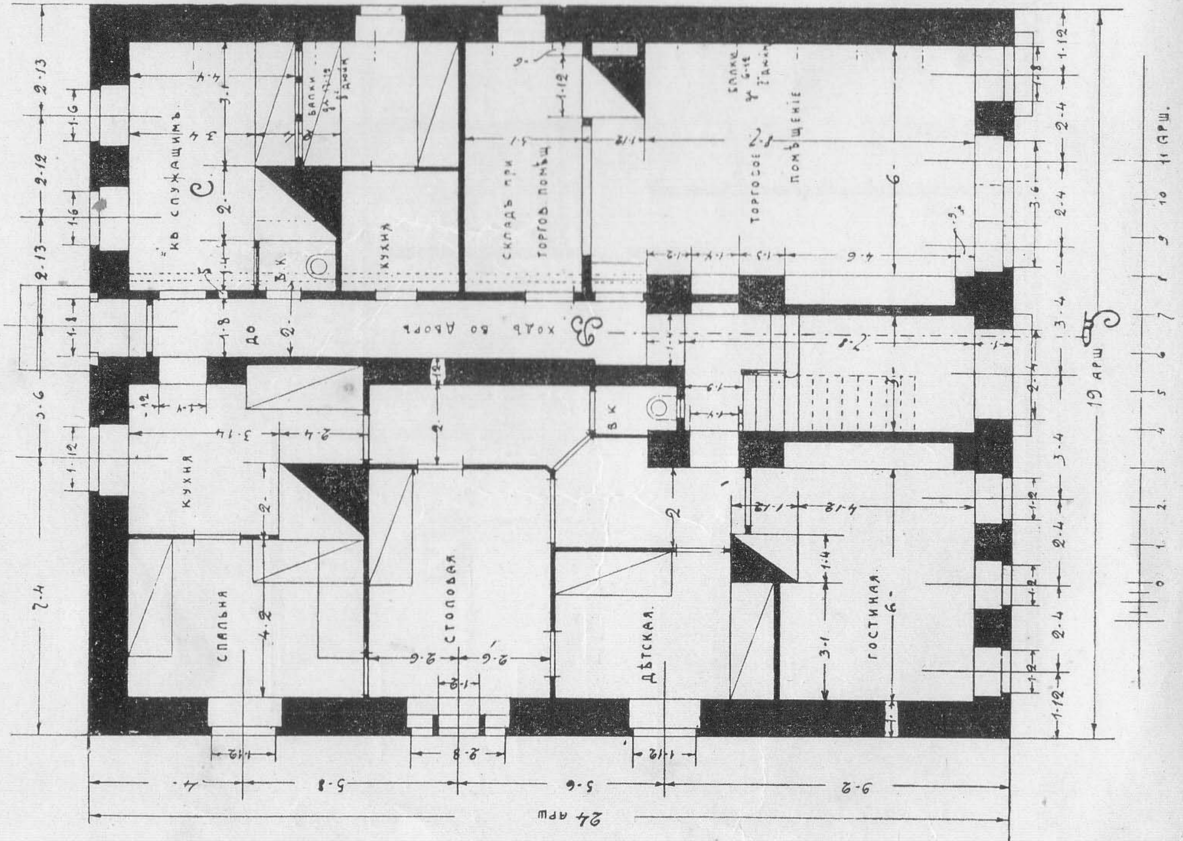
Планъ 1-го этажа.
