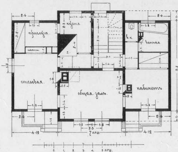
Планъ 2-го этажа.
