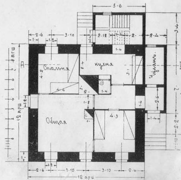
Планъ.
