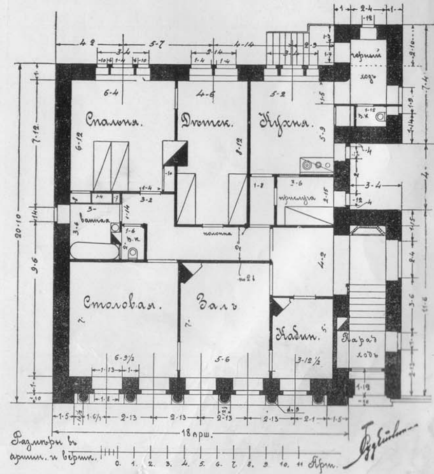
Планъ.
