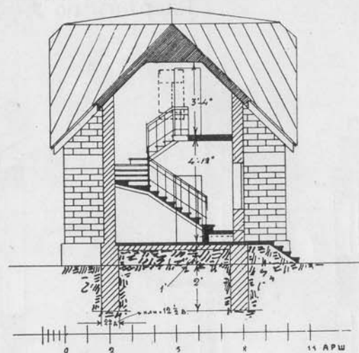
Разрѣзъ по С—Д.
