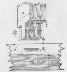
Рис. 150. Замок шиповой простой.
