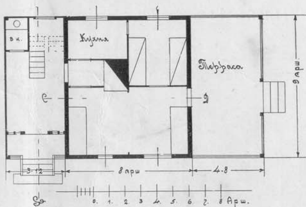
Планъ.
