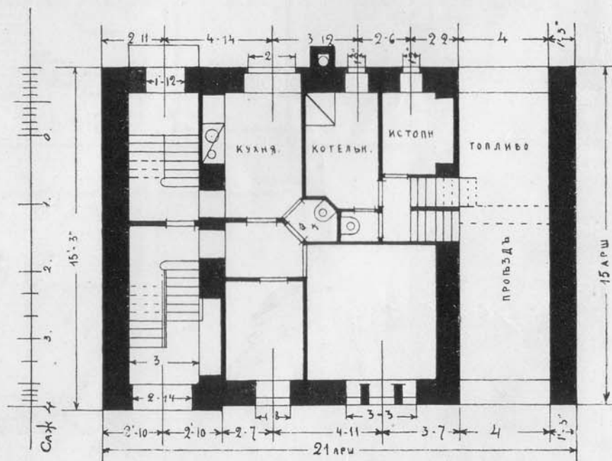
Планъ полуподвала или 1-го этажа*).
