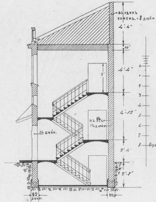
Разрѣзь по лѣстницѣ.
