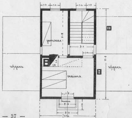
Планъ 2-го этажа.
