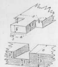
Рис. 145. Замок поперечный въ простой сквородникъ.
