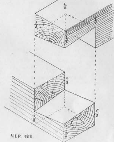
ЗАМОКЪ ВЪ ПОЛОВИННУЮ ЛАПУ.
