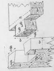
Рис. 144. Замок угловой въ простой сквородникъ.
