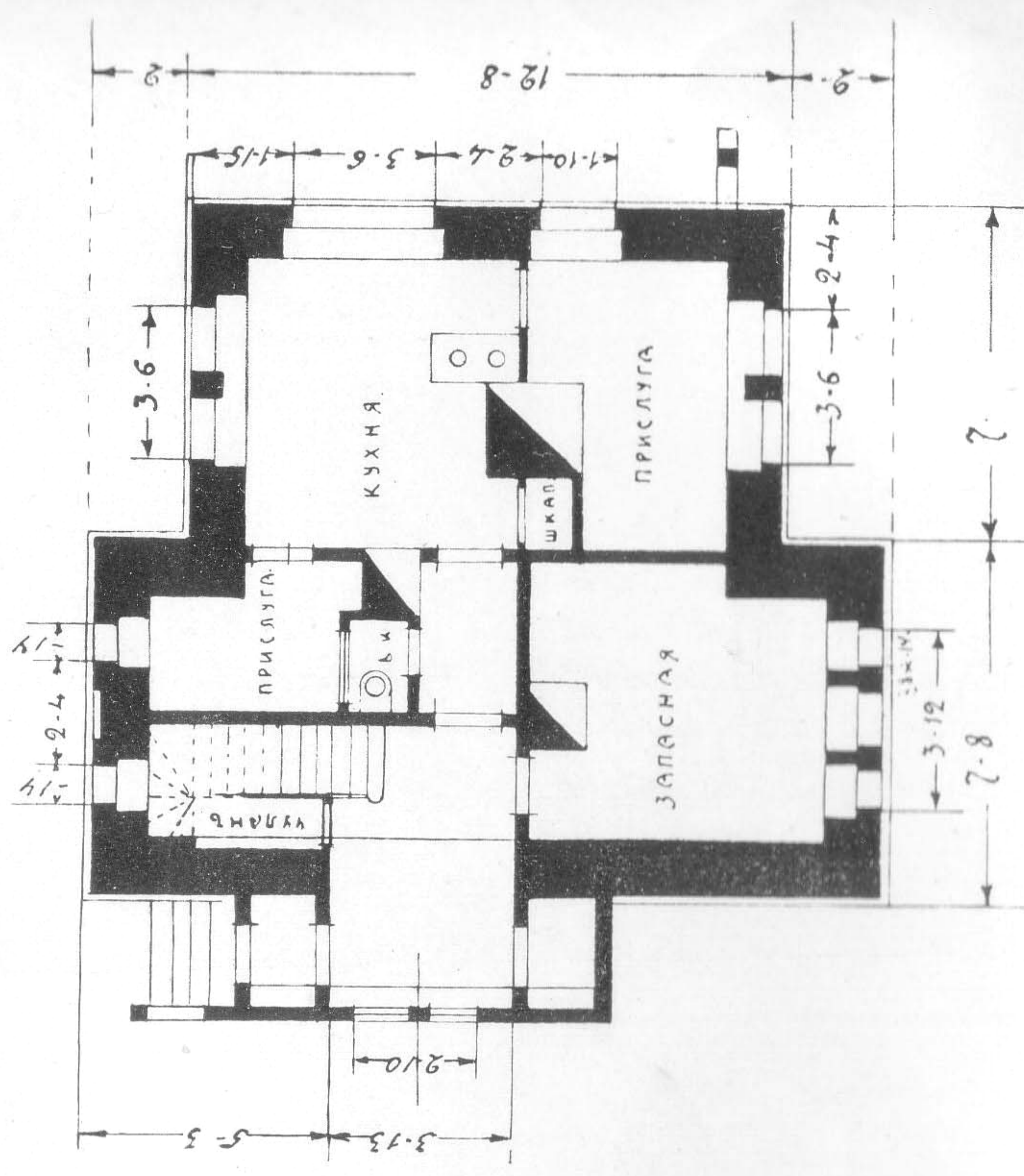
Планъ полуподвала.
