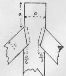
Рис. 166. Замок бабочный с косым зубом и шпиль.
