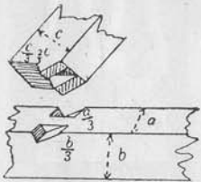
Рис. 162. Косой стропильный замок без шпиль.
