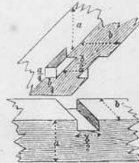
Рис. 148. Замок потемочный нарубной.
