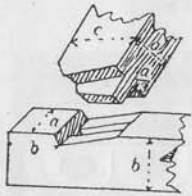
Рис. 155. Стропильный замок с одним зубом и прямым шпиль.
