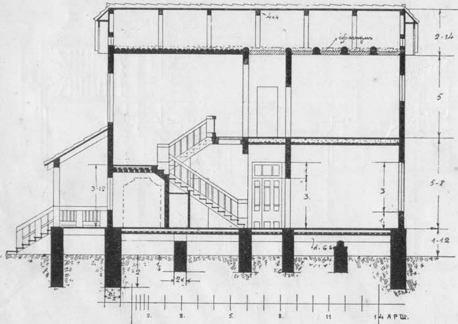
Разрѣзь по С—Д.
