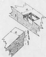
Рис. 147. Замок четвертной двойной.
