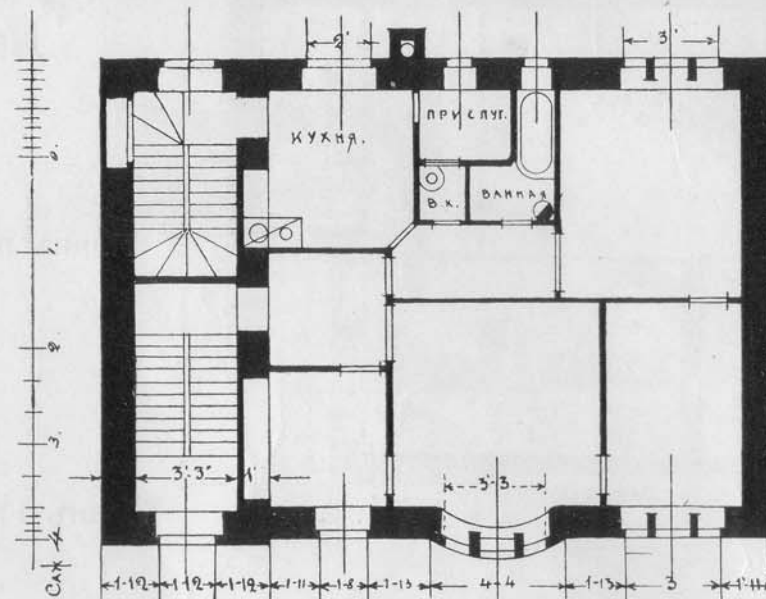
Планъ 2-го, 3-го, 4-го, 5-го этажей.
