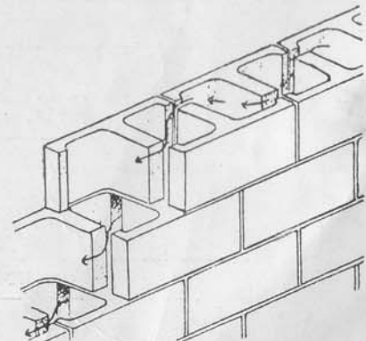
Рис. 196. Т-образный камень.
